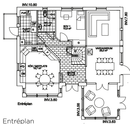
Entréplan
