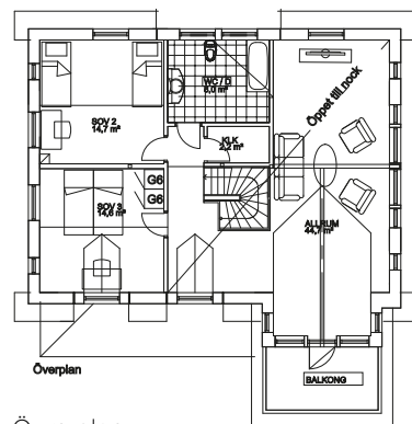
Övre plan
