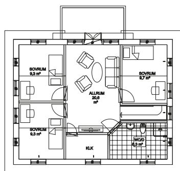
Övre plan
