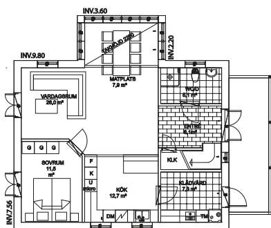
Entréplan
